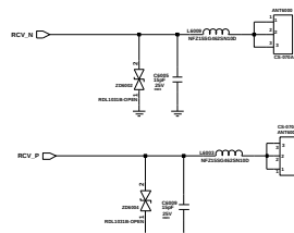
RCV CONTACT
