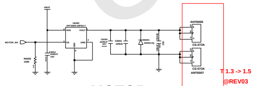
MOTOR
